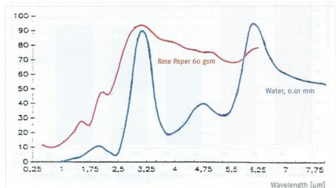
Fig. 2 Absorption du rayonnement IR par une fine couche d'eau et par du papier de base¹.
