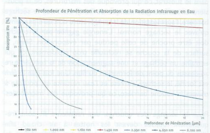
Fig. 5. Profondeur de pénétration et absorption du rayonnement IR par l'eau pour certaines longueurs d'onde des émetteurs à gaz à une profondeur de pénétration de 20 µm.
