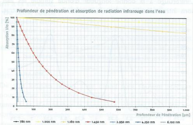
Fig. 4. Profondeur de pénétration et absorption du rayonnement IR par l'eau pour certaines longueurs d'onde des émetteurs électriques conventionnels et optimisés, profondeur de pénétration 1.000 µm.
