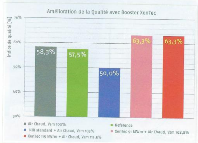
Fig. 7. Amélioration de la qualité par le séchage à partir de la couche de sédiments initiale et la prévention d'un filmage prématuré de la surface.
